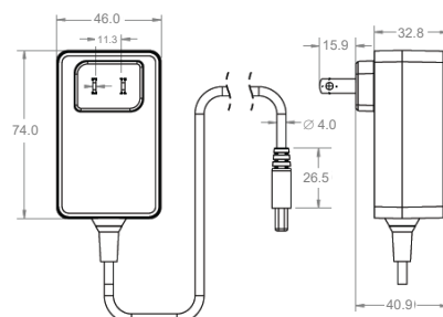
03. ADAPTATEUR DE COURANT - VUE DE L'AVANT ET LATÉRALE
