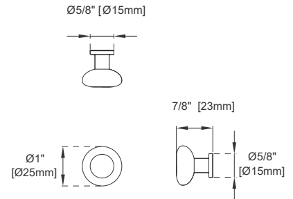
Knob
