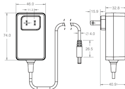
03. ADAPTADOR DE ENERGÍA - VISTA DEL FRENTE Y LATERAL
