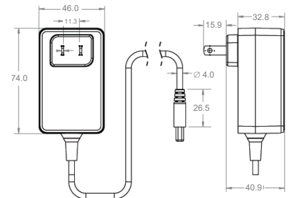
03. ADAPTATEUR DE COURANT - VUE DE L'AVANT ET LATÉRALE
