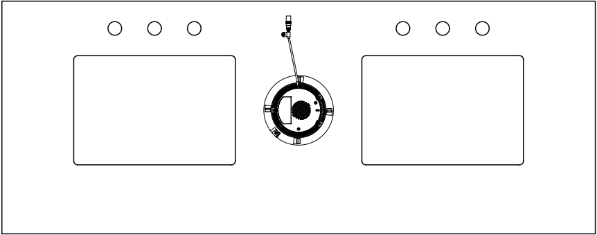
A – Cargador inalámbrico FreePower preinstalado para encimeras de 1.52D m
