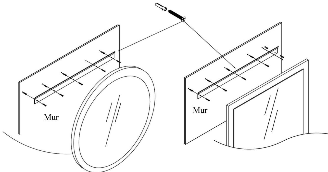
Ancre pour mur creux
