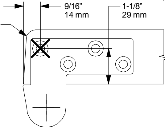
Door Leaf
