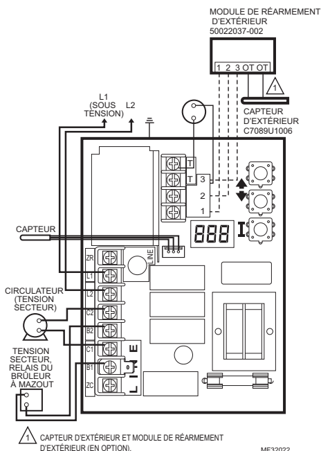
Fig. 8. Connexions à zone unique L7224U.
