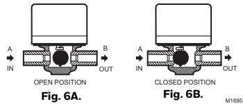
Fig. 6. Valve.
