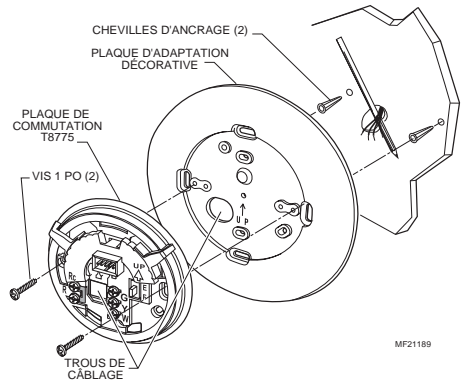
Fig. 1. Montage de la plaque d'adaptation décorative et de la plaque de commutation directement sur le mur (plaque de commutation chauffage-refroidissement illustrée).
