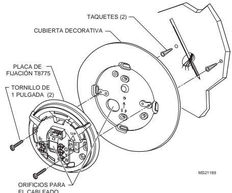
Figura 1. Monte la placa decorativa y la placa de fijación directamente en la pared (se muestra la placa de fijación de calefacción/enfriamiento).
