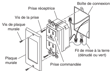
Installation de la prise réceptrice
