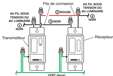
Figure 2 - Câblage de l'interrupteur mural à trois voies
