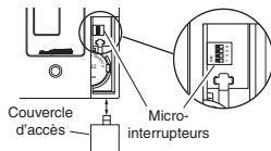
Transmetteur d'appoint
