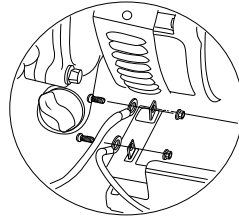
Figure 4-5. Raccordement de la batterie
