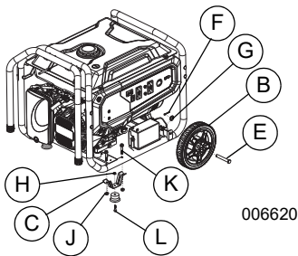
Figura 2-9. Ruedas y patas
