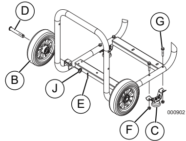
Figure 2-6. Montage des roues et du pied du châssis
