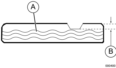
Figura 2-10. Añadir combustible recomendado
