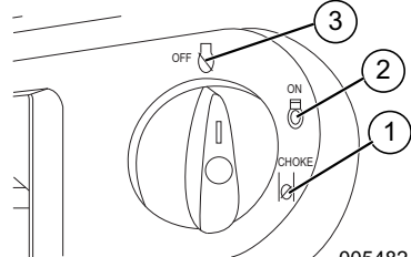
Figure 3-2. Positions OFF/ON/CHOKE (Arrêt/Marche/Étranglement)
