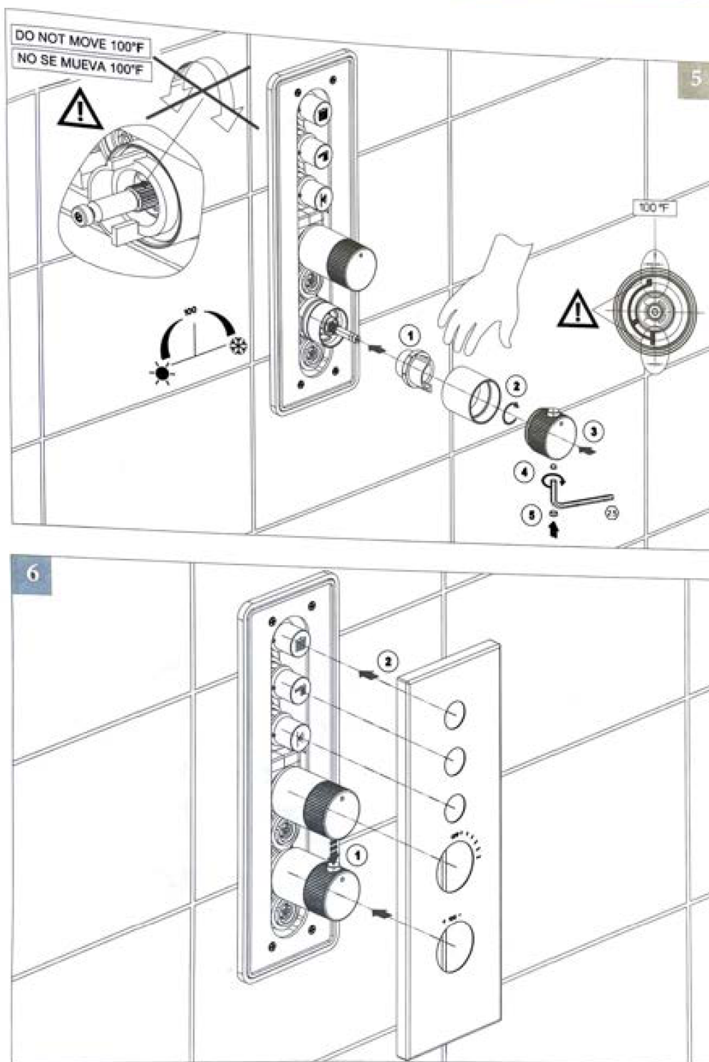
THERMOSTATIC EXTERNAL PARTS - PIEZAS EXTERNAS TERMOSTÁTICAS
