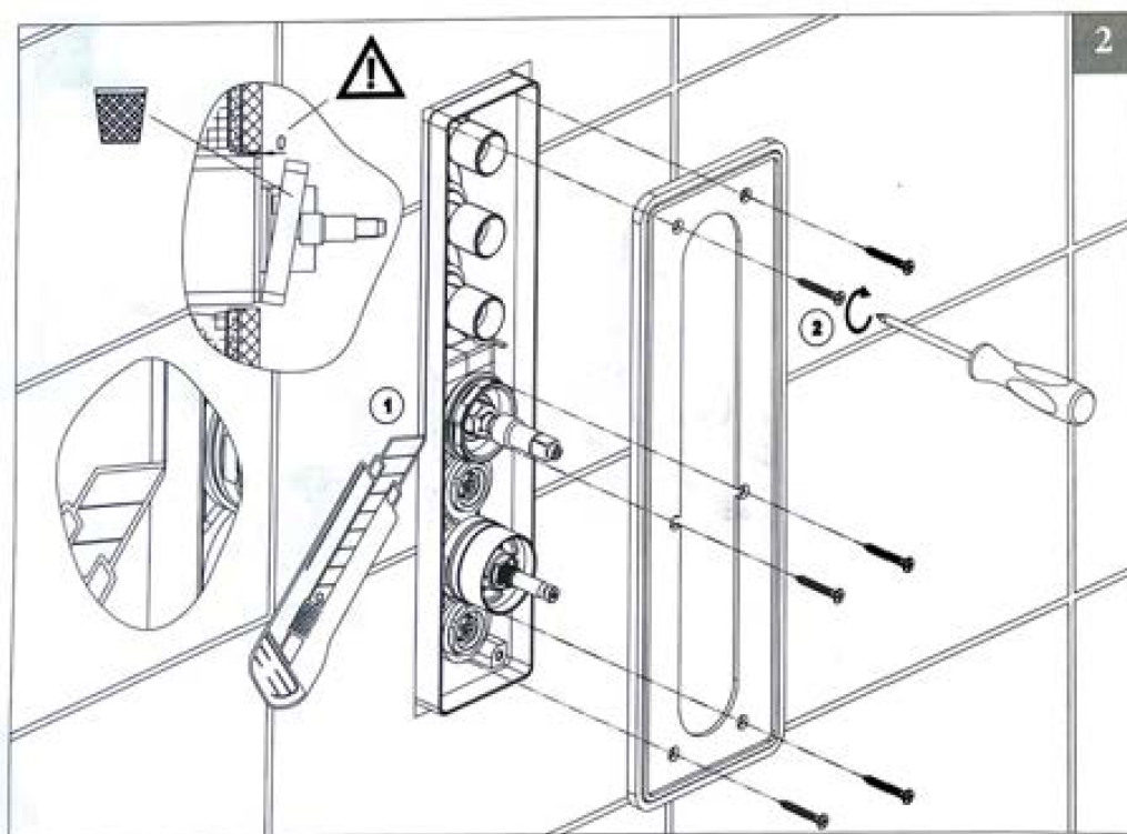
THERMOSTATIC EXTERNAL PARTS - PIEZAS EXTERNAS TERMOSTÁTICAS
