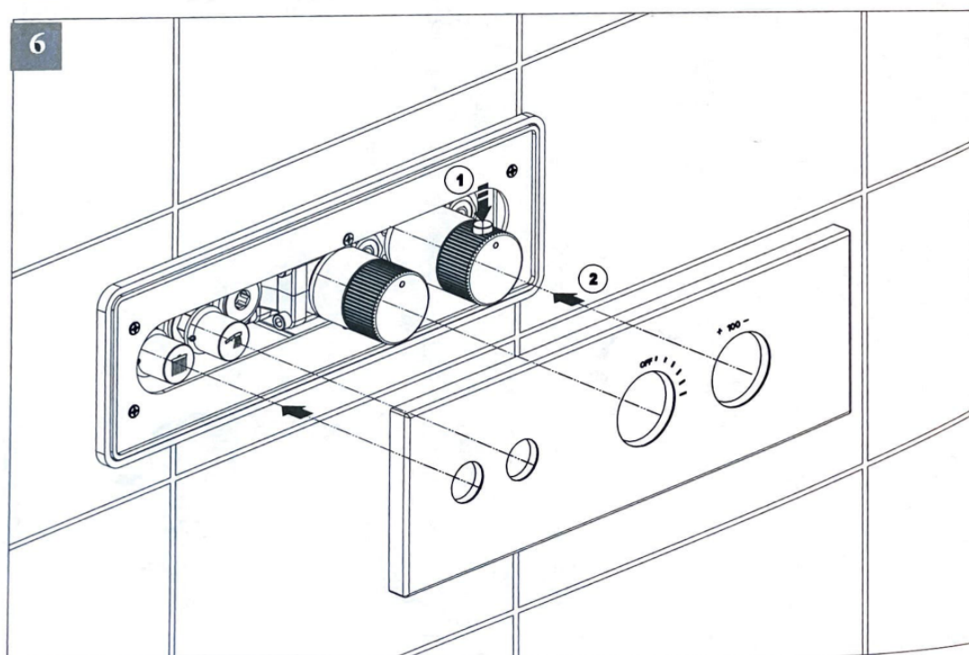
THERMOSTATIC EXTERNAL PARTS - PIEZAS EXTERNAS TERMOSTÁTICAS
