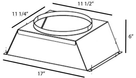
DUCT TRANSITION (for 1200 cfm #IB1200) LA TRASITION DE CONDUIT (pour 1200 cfm #IB1200)
