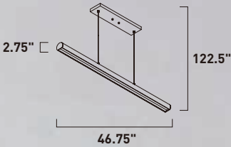
E41467-SA, WT Pendant A
