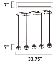
E24257-91PC Pendant
