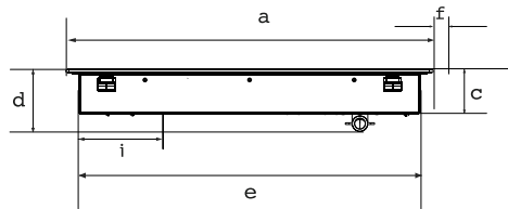
PERFIL
