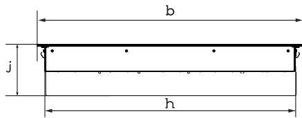
FRONTAL
