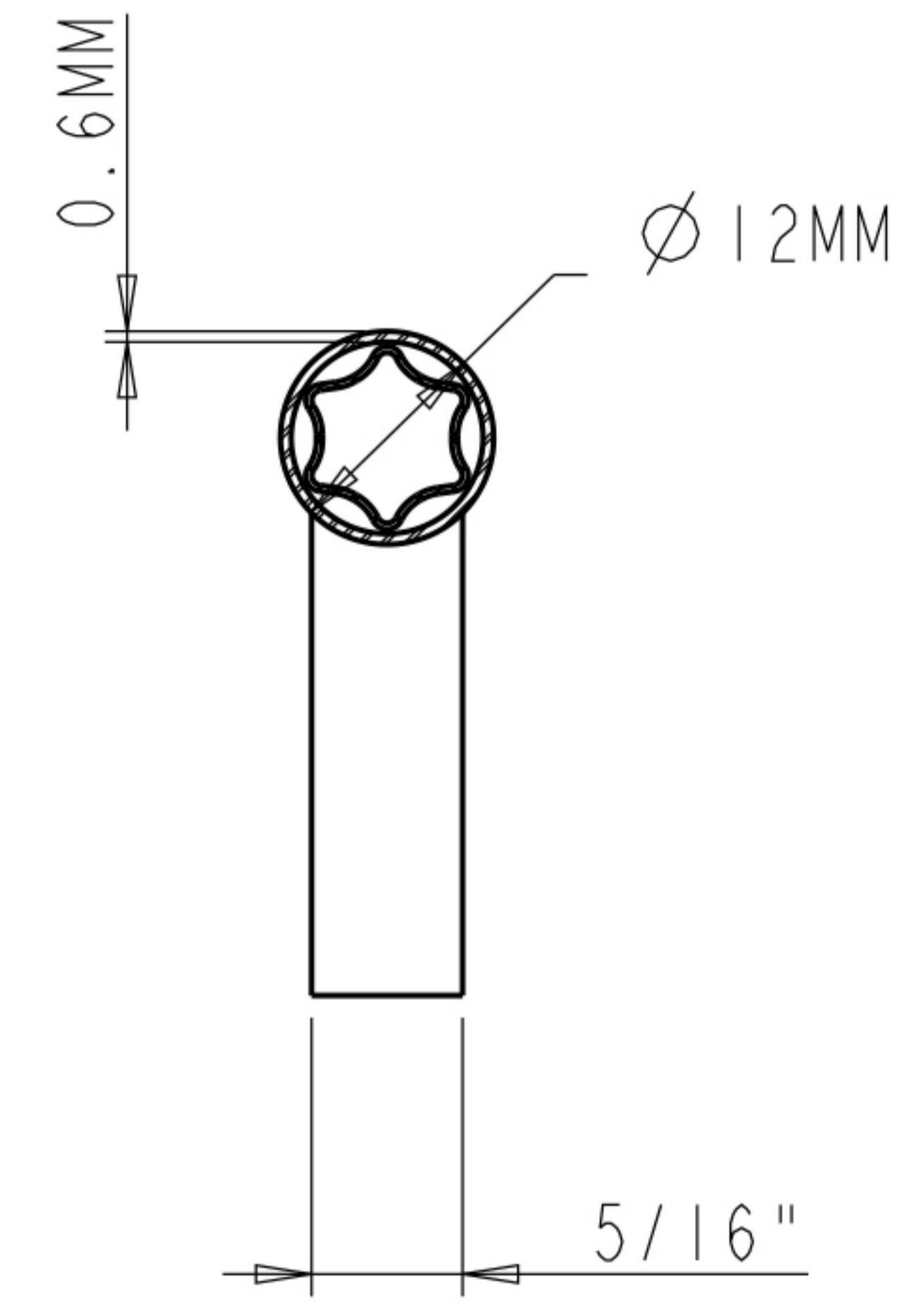
SECTION A-A
