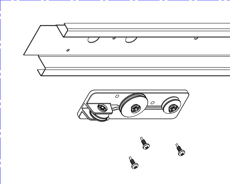
DETTAGLIO A
