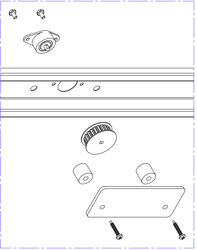
DETTAGLIO B
