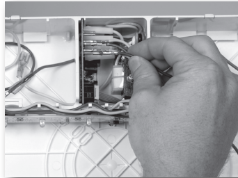
Reconnect lamp leads to the printed circuit board (refer to wiring diagram). Conecte nuevamente los cables de la lámpara a la placa de circuitos impresos (consulte el diagrama del cableado).
