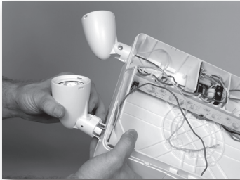
Route lamp leads through new hole location and press fit lamphead into new location. Canalice el cable de la lámpara por el nuevo agujero y presione la cabeza de lámpara en el nuevo lugar.
