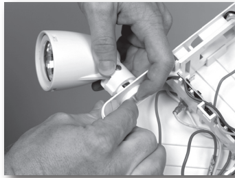
Remove lamphead from housing by squeezing press fit tabs from inside of housing. Retire la cabeza de lámpara de la caja presionando las pestañas desde el interior de la caja.
