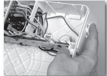
Press fit hole plug into old lamphead hole location. Presione el tapaagujeros en el lugar que quedó libre después de retirar la cabeza de lámpara.
