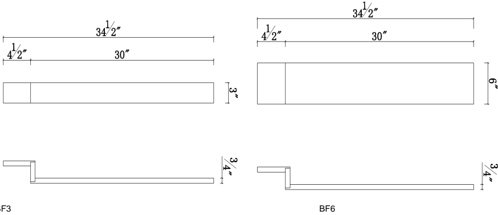
BF3
