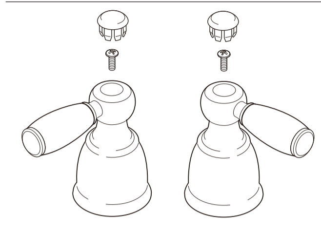
RP42995 ▲ Hot & Cold Lever Handles w/Buttons & Screws Manijas en Palanca con Botones y Tornillos de agua fría y caliente Manettes-levers d'eau chaude et d'eau froide avec boutons et vis
