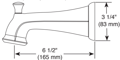
RP52153 ▲ (Pull-Up Diverter)
