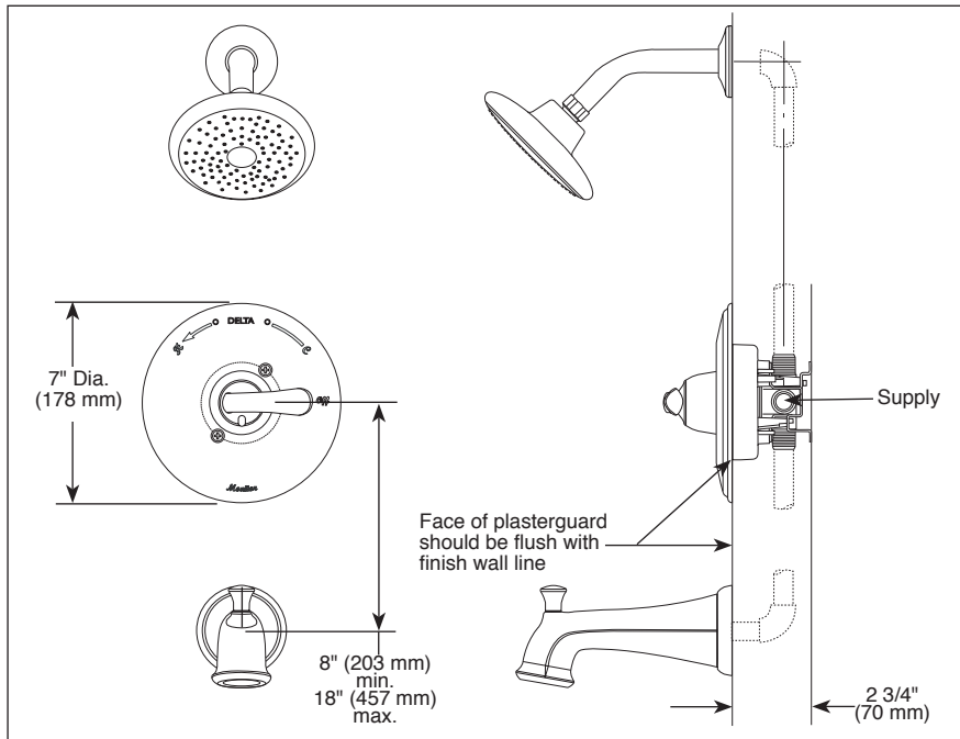
RP54752 ▲ 1.5 GPM H 2 O Showerhead
