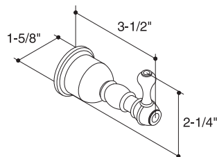
Robe Hook
