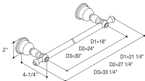
18", 24", 30" - Towel Bar
