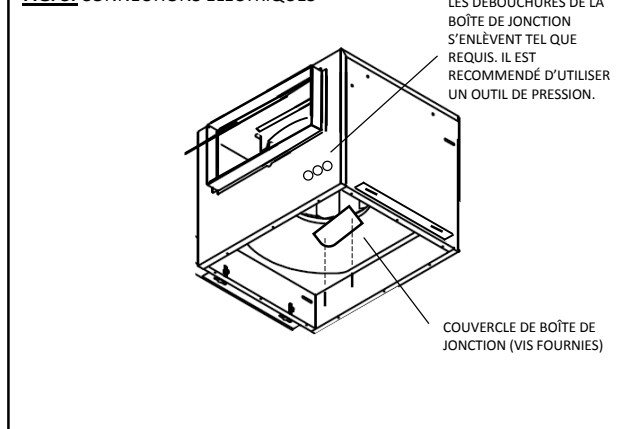
FIG. 3: CONNECTIONS ÉLECTRIQUES
