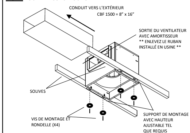
FIG. 1: NOUVELLE CONSTRUCTION
