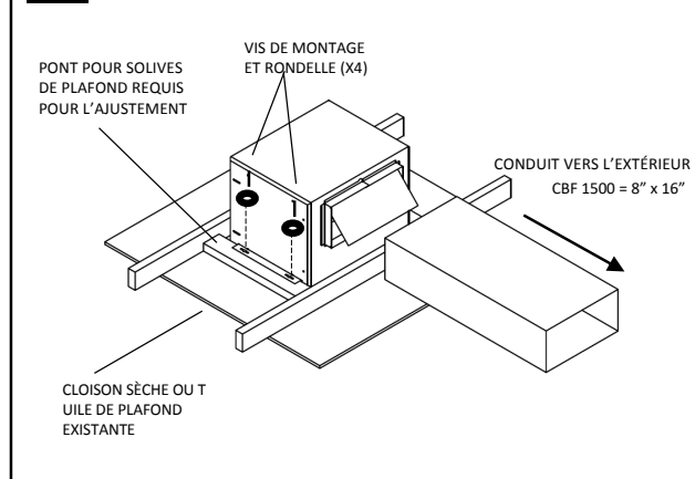
FIG. 2: CONSTRUCTION EXISTANTE MODIFIÉE
