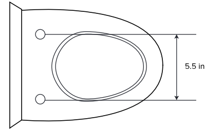
Distance Requise Entre les Boulons de Montage
