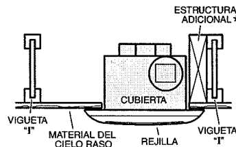
CUBIERTA MONTADA EN UNA VIGUETA "1" Se requiere una estructura adicional para el montaje. Descarga paralela a las viguetas.
