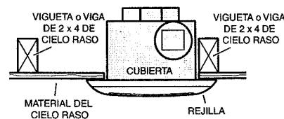
CUBIERTA MONTADA DIRECTAMENTE EN LA VIGUETA 2 X 6 Descarga paralela a las viguetas.
