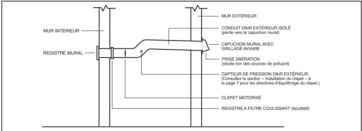
Clapet et conduit extérieur raccordés directement au registre d'un plafond, d'un mur ou d'un plancher.
