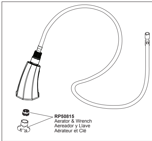
RP84357▲ Hose & Sprayer Assembly Ensamble de la tubería y rociador Tuyau souple et douchette
