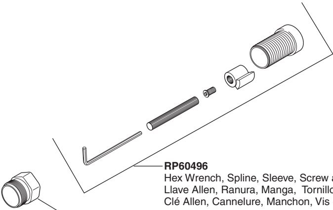
RP54912 Bonnet Nut Bonete Chapeau Fileté
