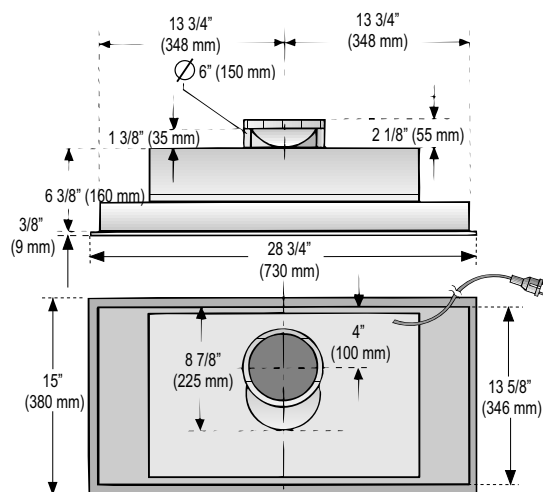
Figure 6: Dimensions générales - modèles de 28 7/8 po (73 cm)
