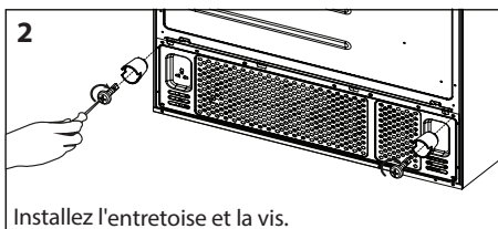
2 Installez l'entretoise et la vis.
