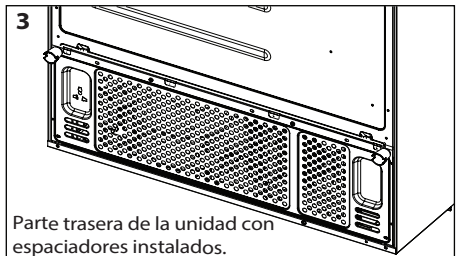
Instale el espaciador y el tornillo.
