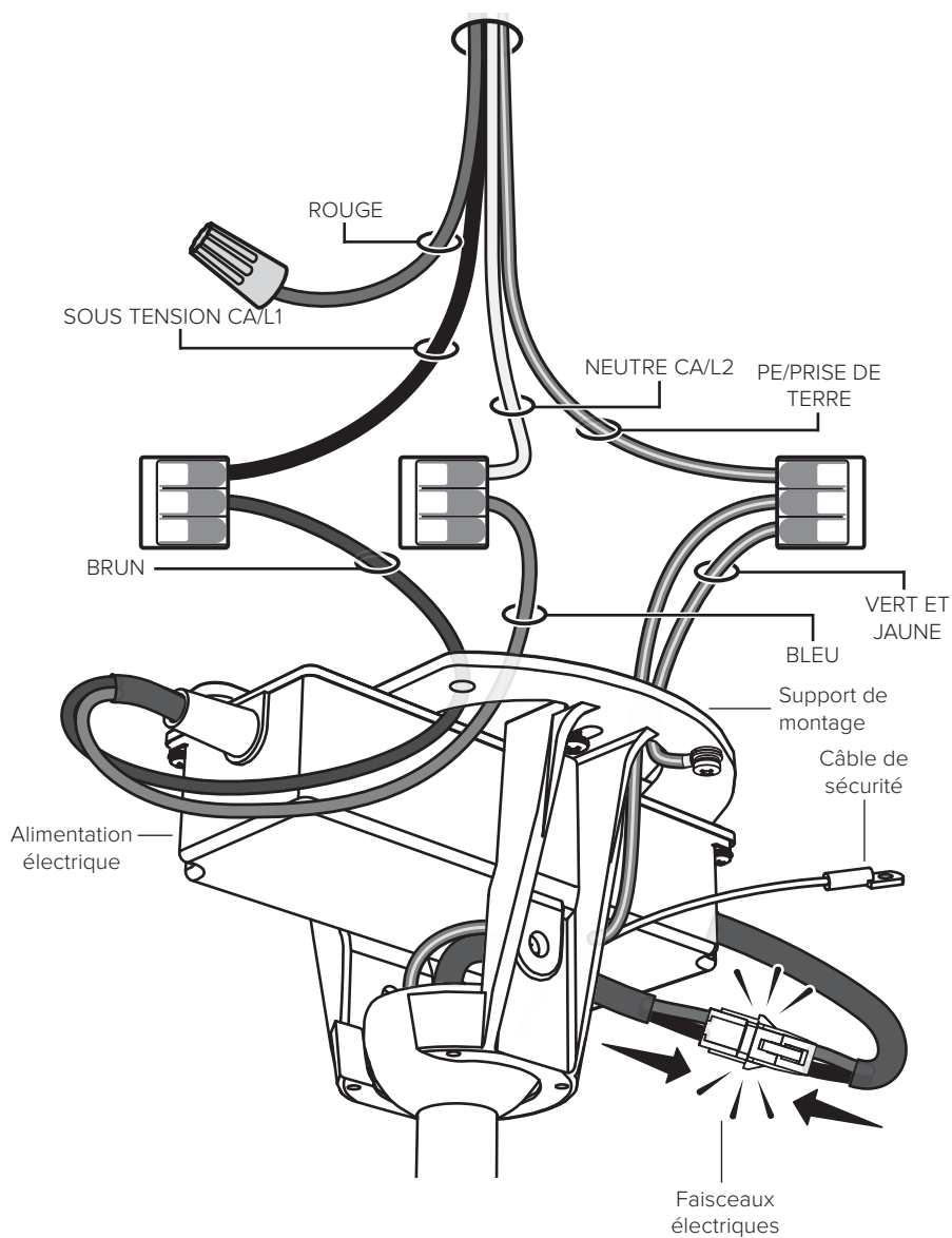
Fig. 11a : Diagramme de câblage (sans filtre EMI)
