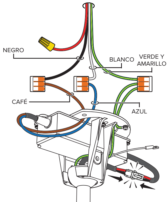
Diagrama de cableado (Sin filtro EMI)
