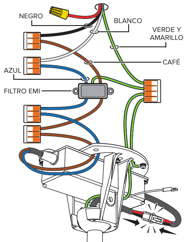
Diagrama de cableado (Con filtro EMI)
