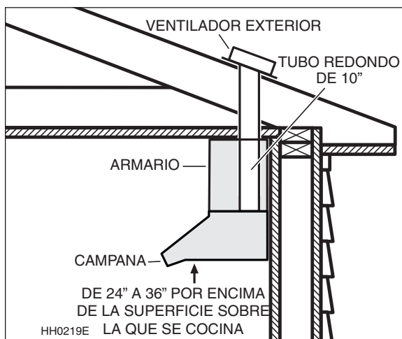
INSTALACIÓN HABITUAL CON VENTILADOR EXTERIOR EB6, EB9, EB12 O EB15
