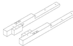
B x2 Headboard Legs (Left & Right) * x2 Pattes de la tête de lit (gauche et droite) x2 Patas de cabecera (izquierda y derecha)
