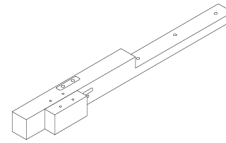
x1 RP166160-LEGL-Left Leg * Patte de gauche Pata izquierda
