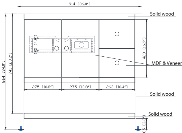
Front / Devant
