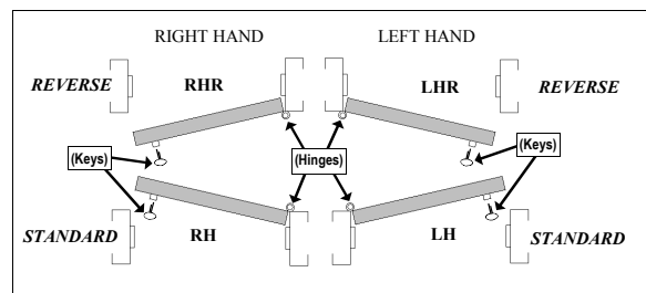
Fig. 2: Cross Section Top View -- Door Hand
