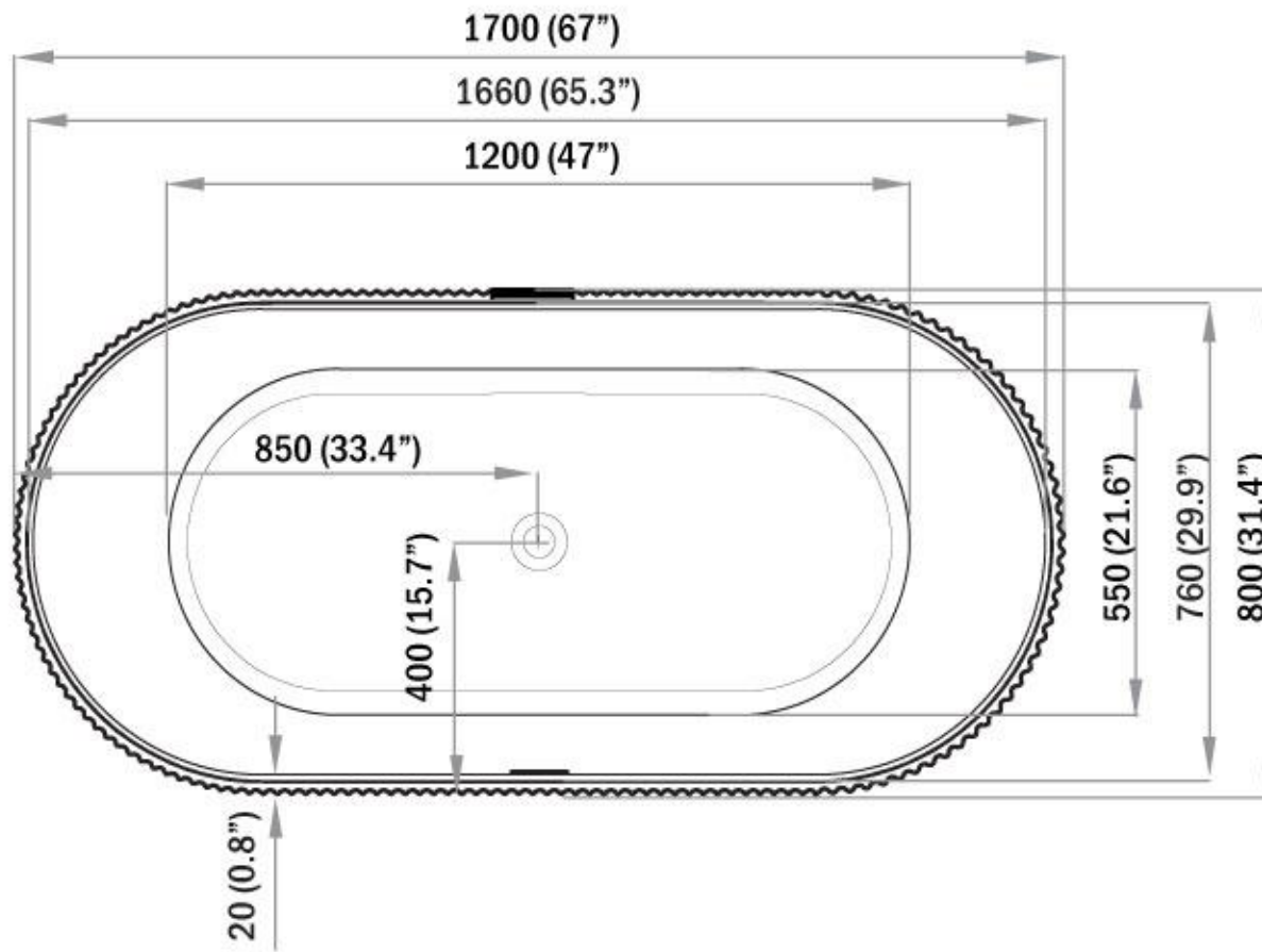
TOP VIEW -VUE DE DESSUS
