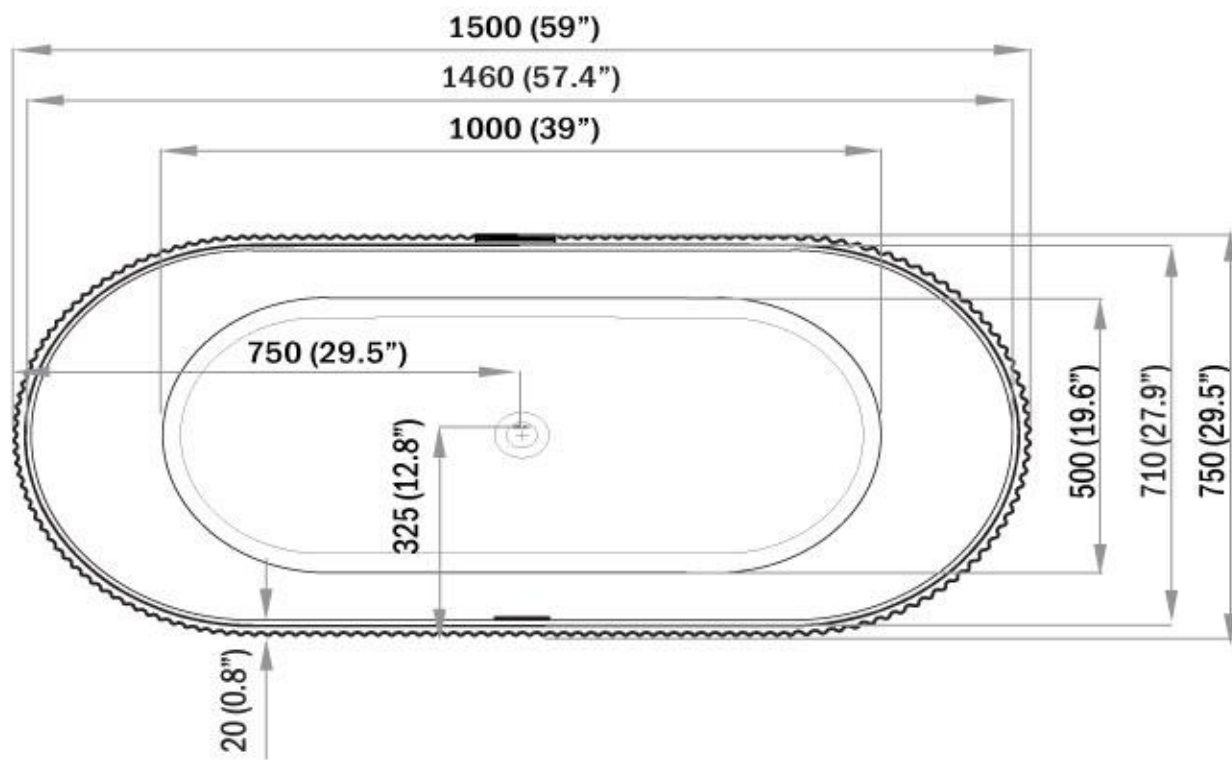
TOP VIEW -VUE DE DESSUS
