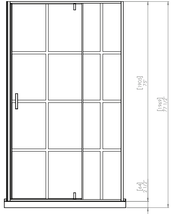
FRONT VIEW VUE DE FACE
