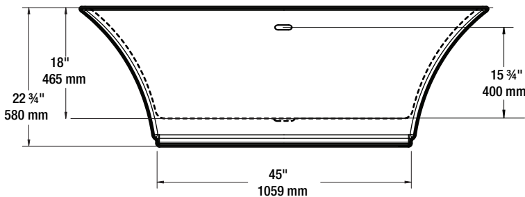
FRONT VIEW VUE DE FACE
