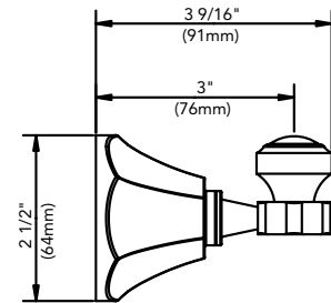
ROBE HOOK
