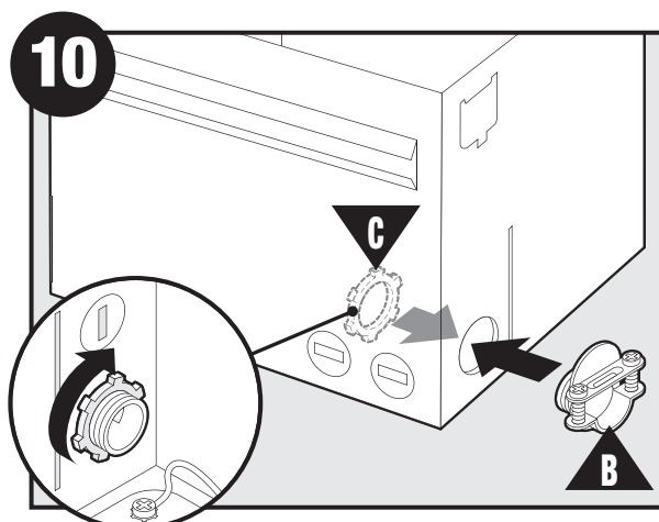
10 Introduire le raccord (non compris) dans le boîtier et le fixer avec une rondelle.
