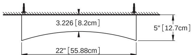
Vista superior
