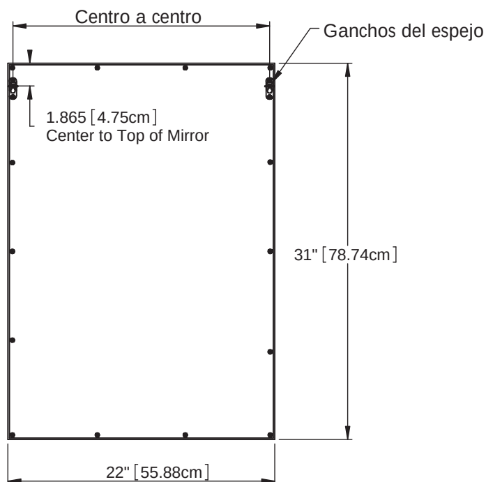
Vista posterior
