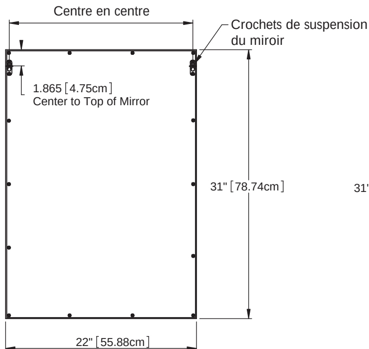
Vue arrière
