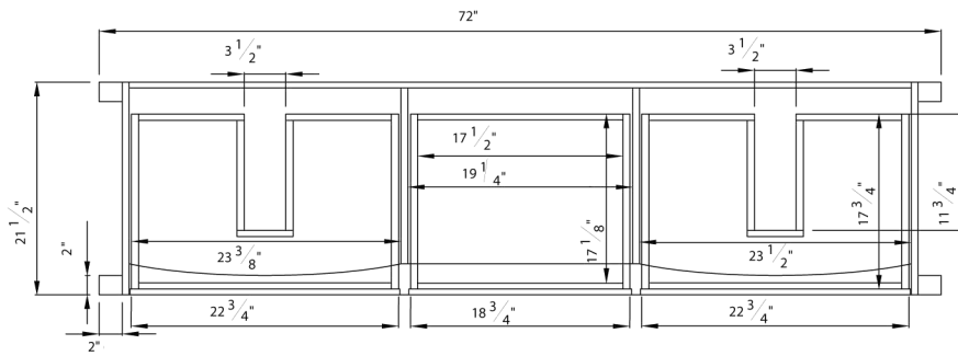
TOP
