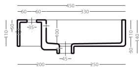
Sezione longitudinale
