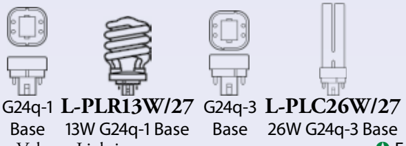
G24q-1 L-PLR13W/27 Base 13W G24q-1 Base G24q-3 L-PLC26W/27 Base 26W G24q-3 Base
